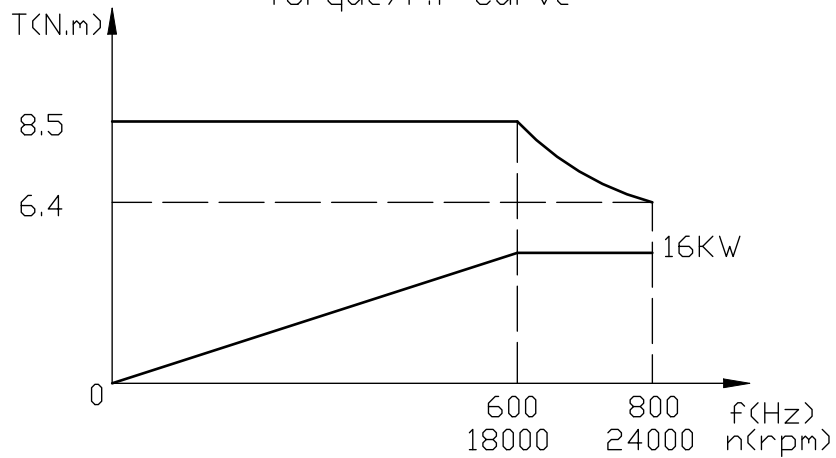
扭矩/功率曲线
