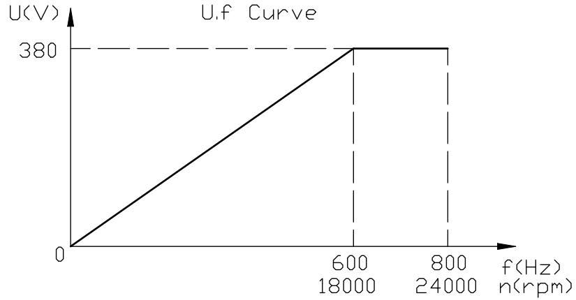
频压曲线
