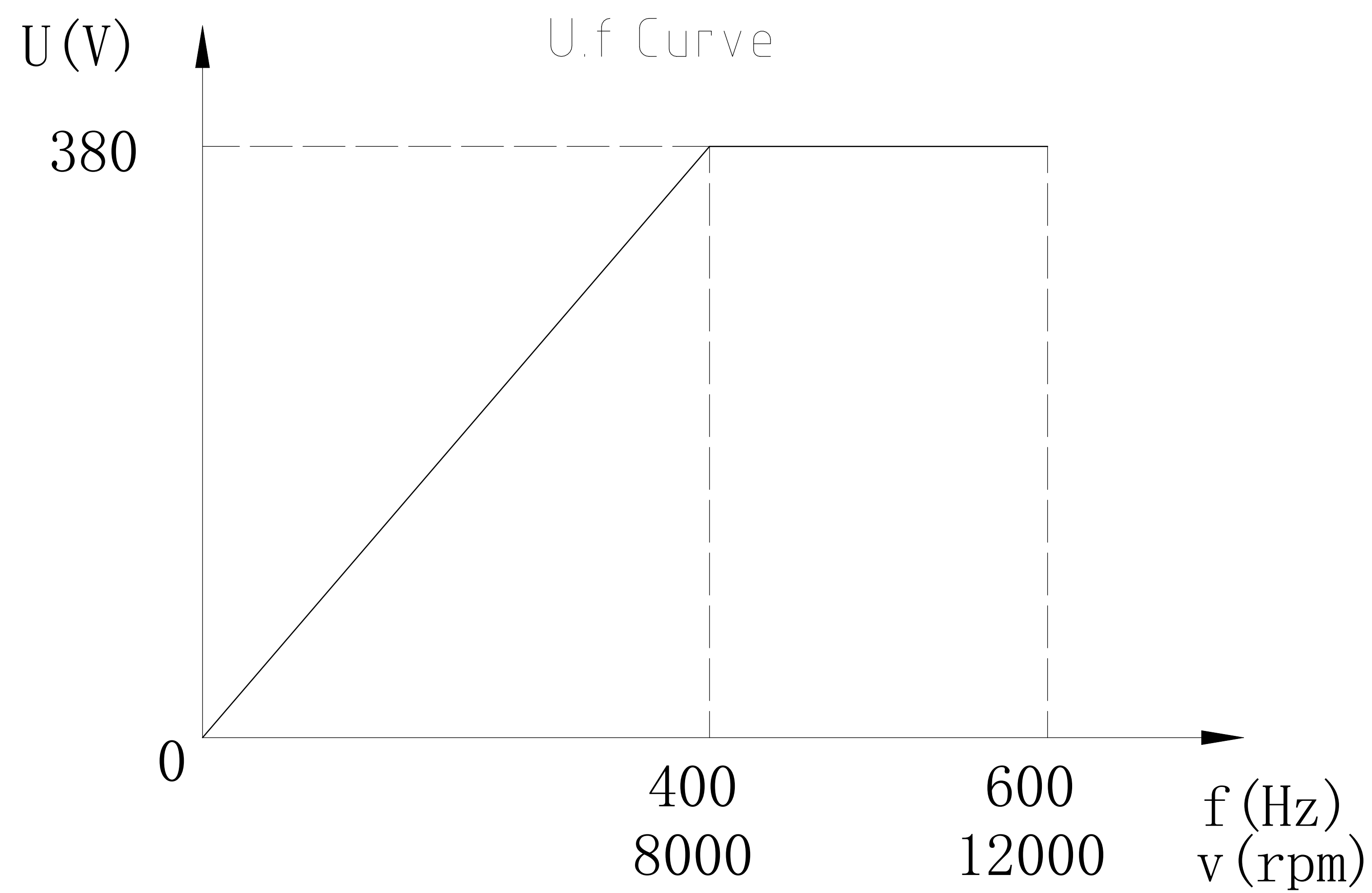
频压曲线
