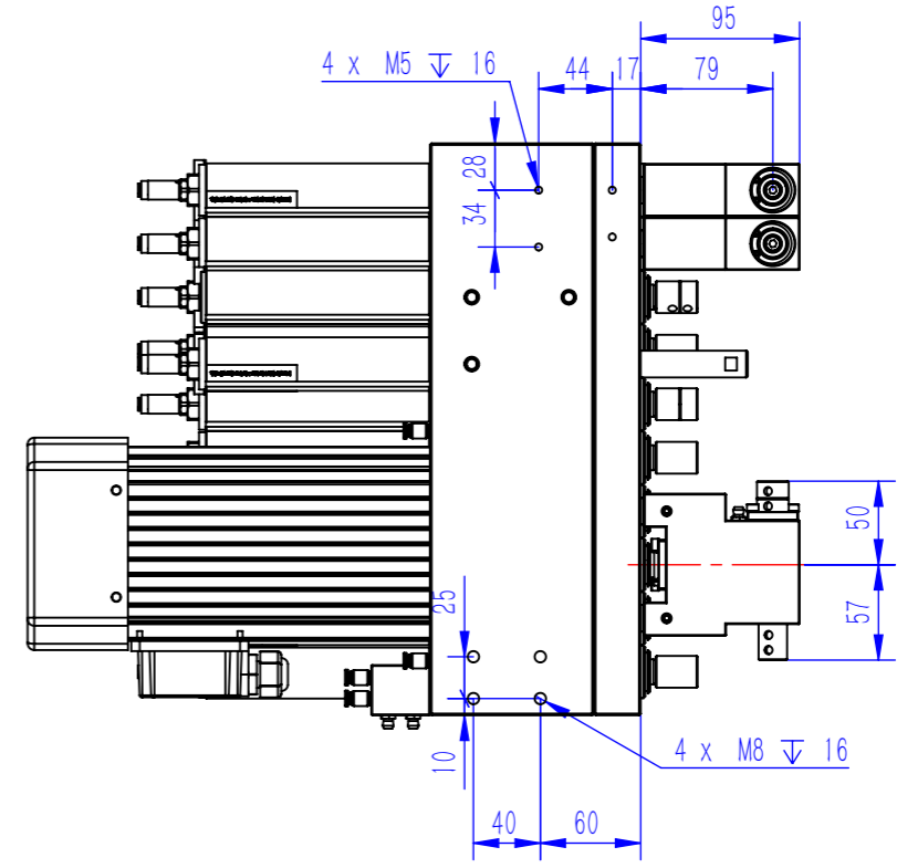
视图 B
