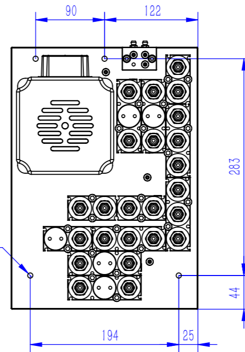
视图 B
